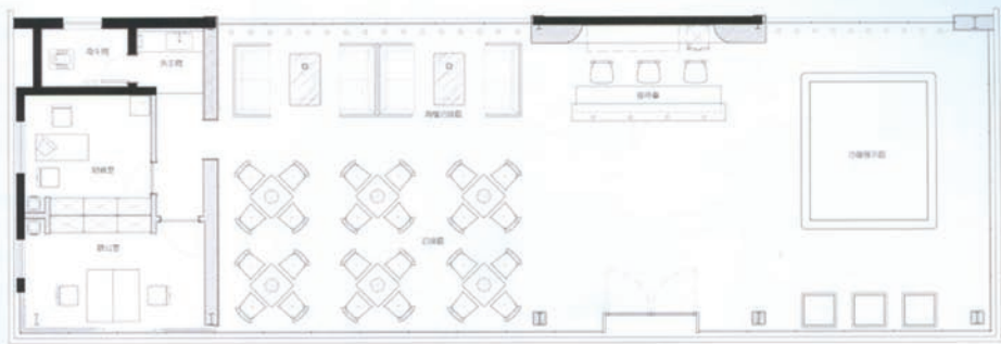
平面布置图
